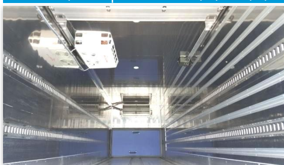
F4 : 2채널 Evaporator + 칸막이 + 히터
